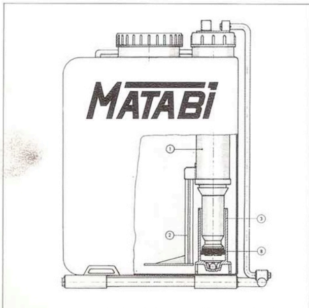
Corte del modelo SUPER
